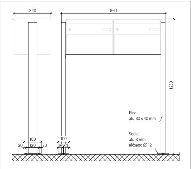
Support latéral avec profilé en U supplémentaire avec plaque de base
