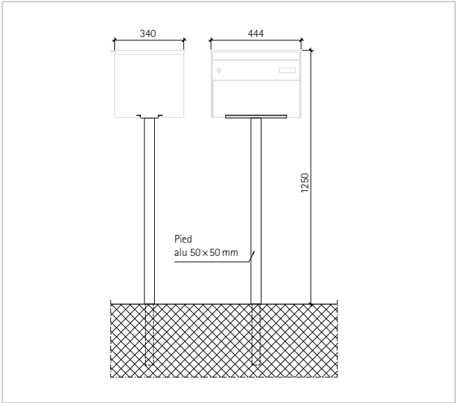
Support latéral avec plaque de base
